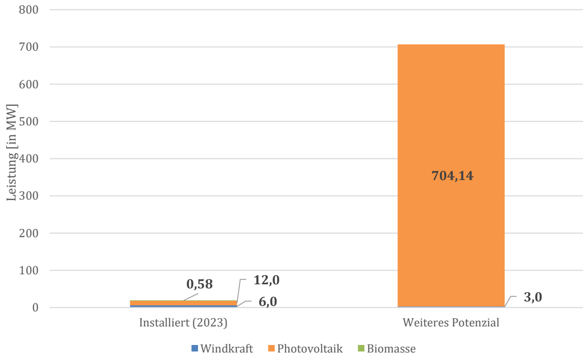
Abbildung 4: Installierte und offene, potenzielle Leistung der erneuerbaren Energieanlagen [5-8]
